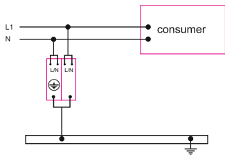
Еднофазна TT система
