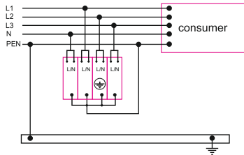
Трифазна TN-S система
